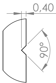
SZCZEGÓŁ A SKALA 5 : 1
